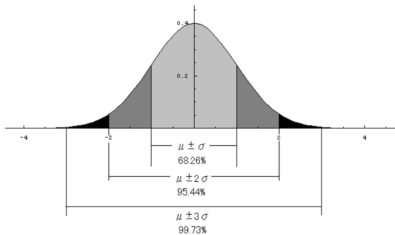
図 9 正規分布の性質
