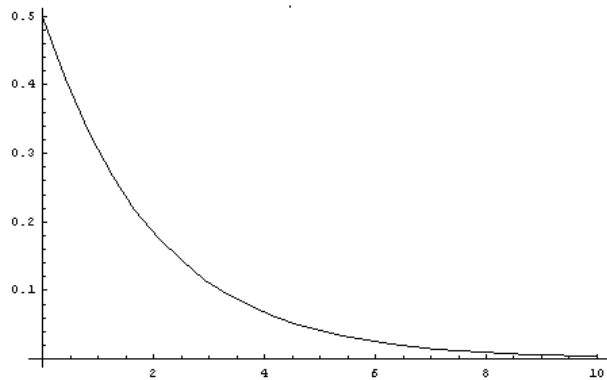
図 11 二つの二乗標準正規分布を足した分布
