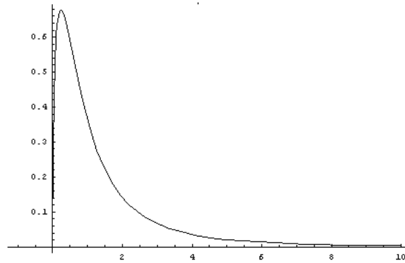
図 15 F(3, n) の分布
