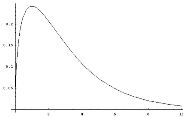
図 12 三つの二乗標準正規分布を足した分布
