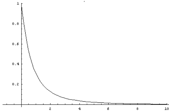
図 14 F(2, n) の分布
