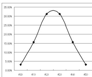
図 1 普通のコインの確率関数は対称型
