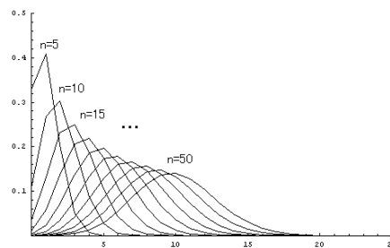
図3 いびつコインでも反復すると
