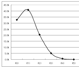
図2 五回に一回しか表が出ないコインでは
