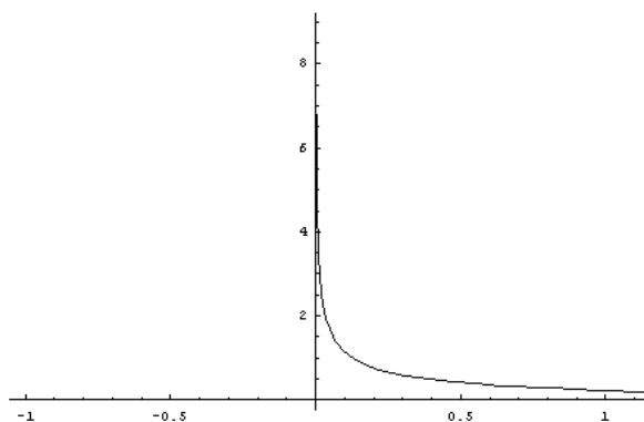
図 13 F(1, n) の分布
