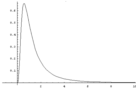
図 16 F(10, 5) の分布
