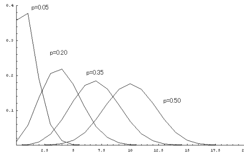
図4 様々なコインを試してみると
