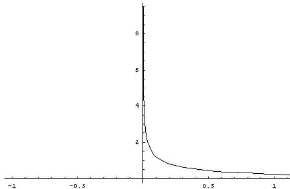
図 10 標準正規分布を二乗した確率変数の分布
