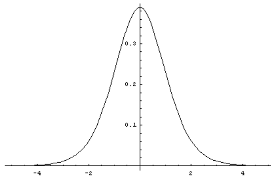
図 17 自由度 10 の t 分布
